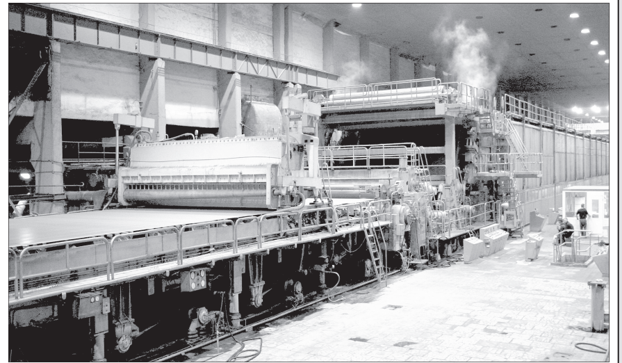
Вторая картоноделательная машина производства картона АЦБК
