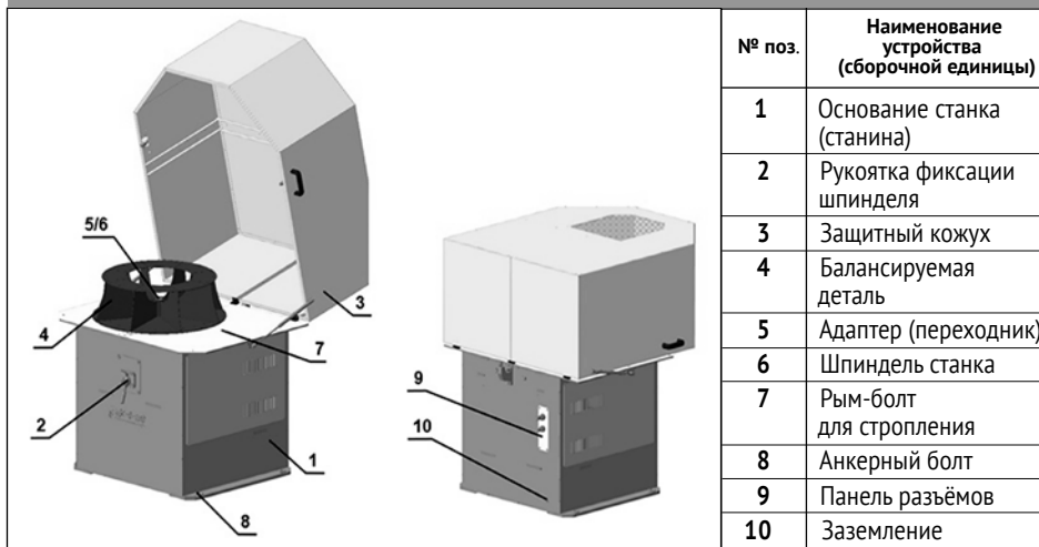
Внешний вид и составные части балансировочного станка БС-В-200
